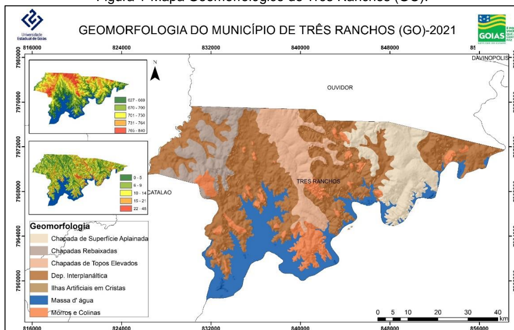
Figura 1-Mapa Geomorfológico de Três Ranchos (GO).
