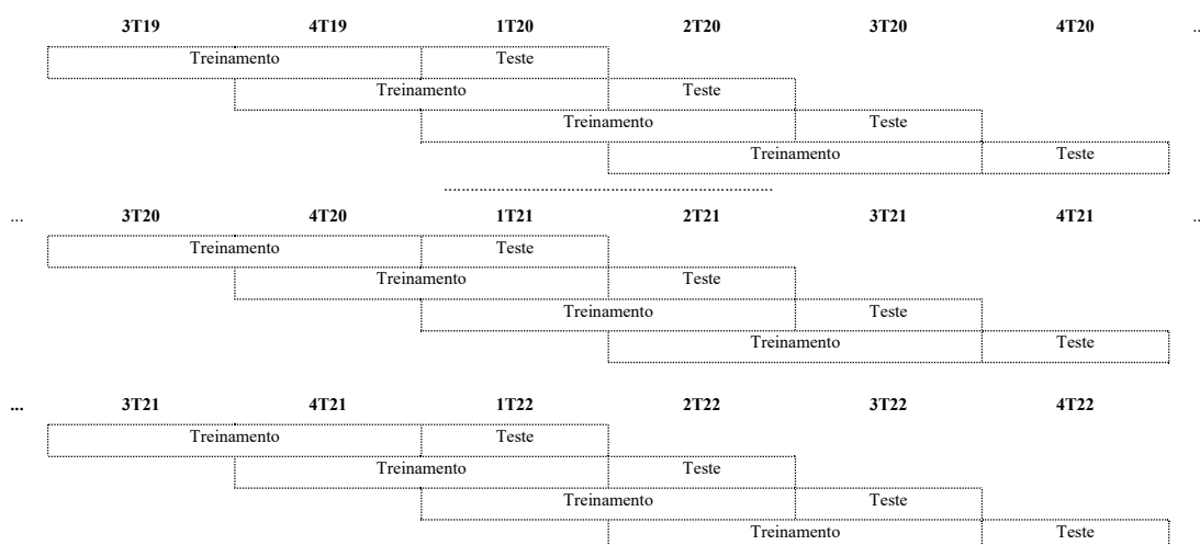
Figura 2. Divisão da base de dados nos 12 distintos conjuntos de treinamento/teste
