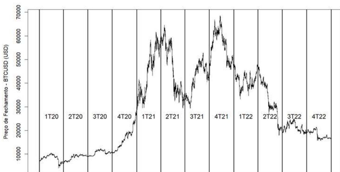
Figura 3. Evolução do preço de fechamento intradiário do Bitcoin no período de janeiro de 2020 a 2022. A linhas horizontais indicam a divisão dos períodos pelos 12 trimestres de amostras teste.
