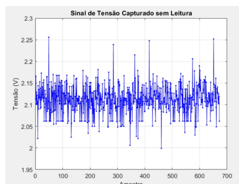
Graph 1. Sinal de tensão em repouso usado para medir o desvio padrão do ruído real.
